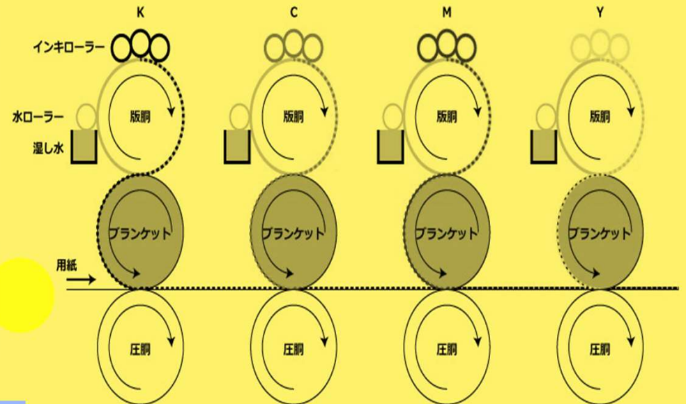
<オフセット印刷の仕組み>
