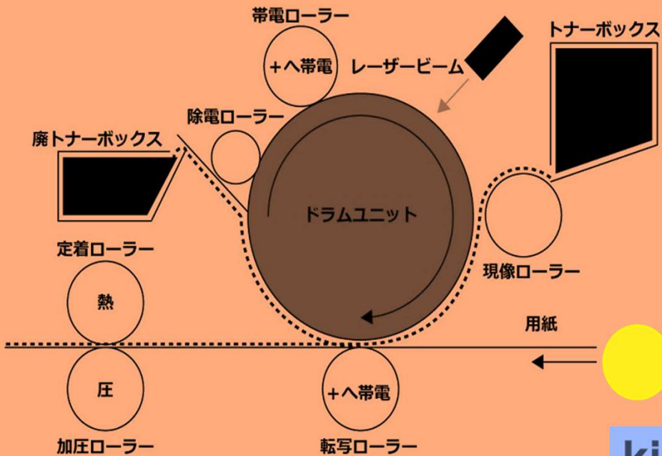
<オンデマンド印刷（レーザープリント）の仕組み>
